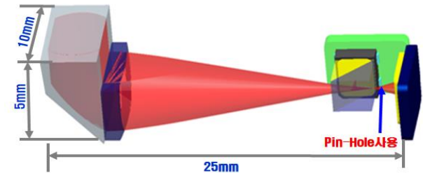
광학식 Module Structural Diagram
